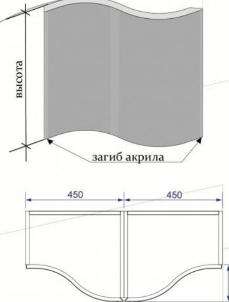
S-образный фасад вариант №2 (выпуклый)
