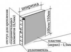
Цоколь
