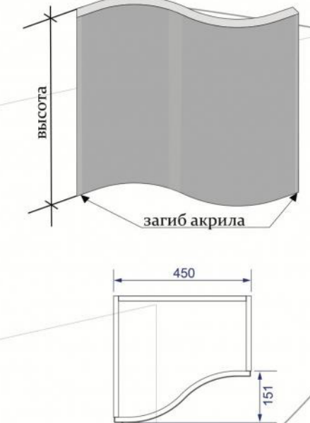
S-образный фасад вариант №3 (выдвижной ящик)
